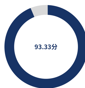
图 3：平均得分
